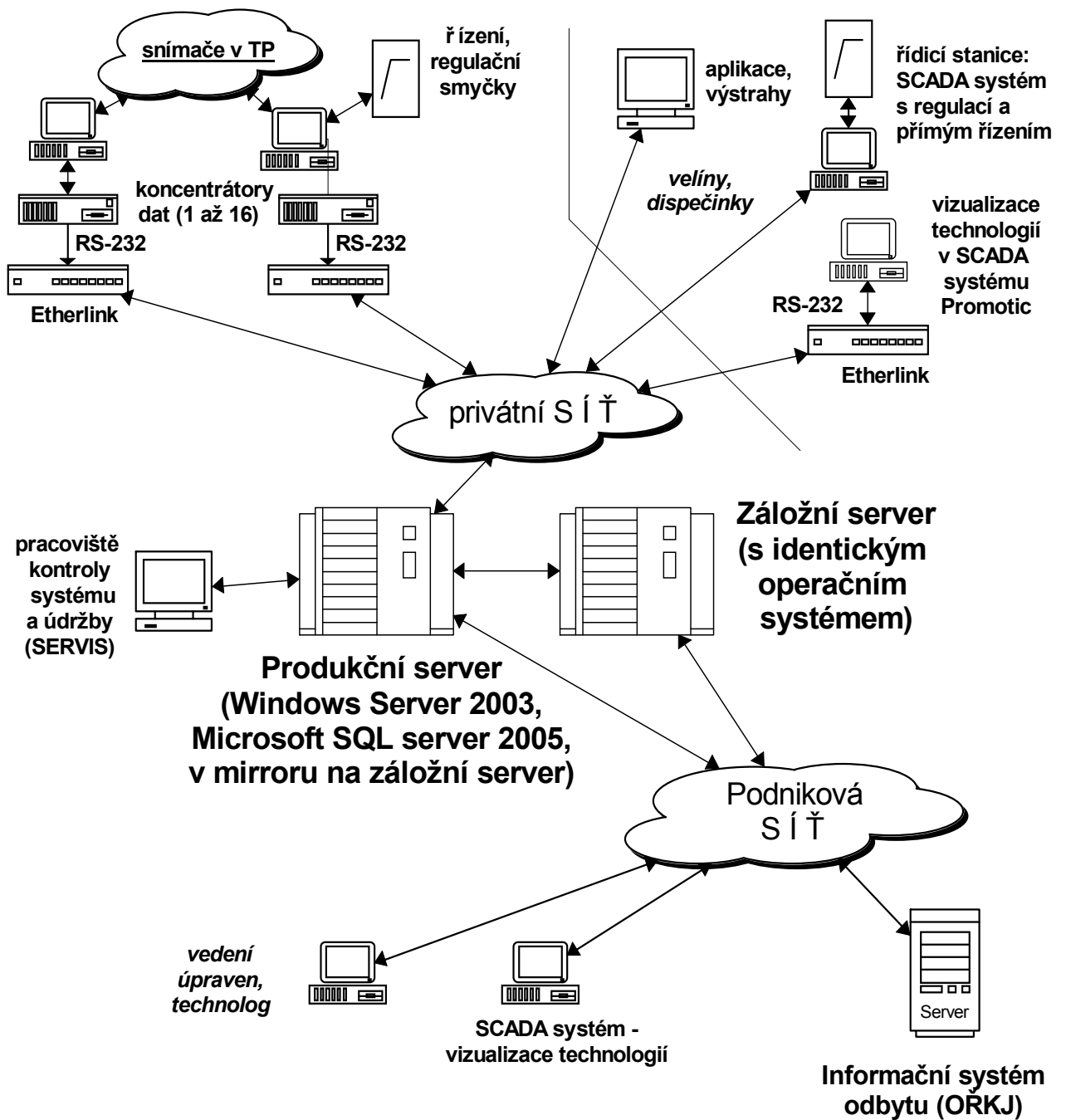
Schéma řídicího systému úpravny KOVIS
